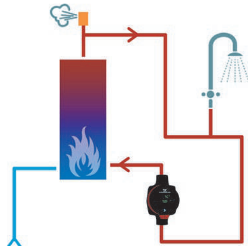
Abb. 6 Häusliches Warmwasserzirkulationssystem
