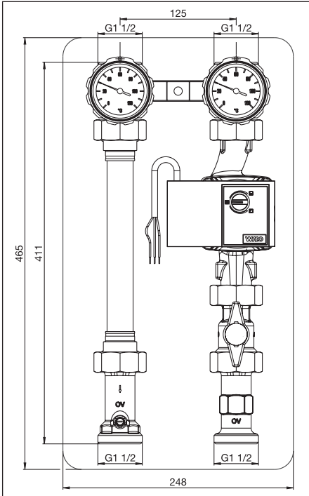
Fig. 3 Système de raccordement pour chaudières 180 mm DN25 avec robinet d'isolement à tournant sphérique (forme longue)
