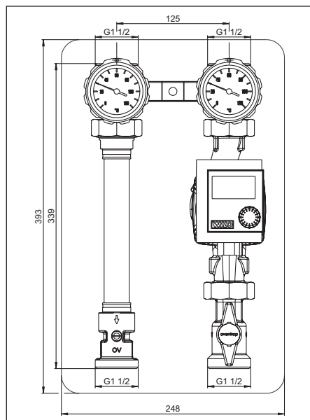
Fig. 5 Système de raccordement pour chaudières 180 mm DN25 avec robinet d'isolement à tournant sphérique (forme courte)
