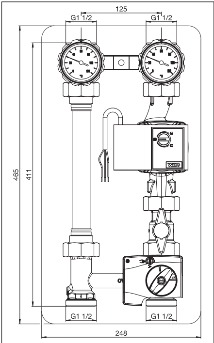
Fig. 4 Système de raccordement pour chaudières avec vanne mélangeuse à trois voies 180 mm DN 25 avec robinet d'isolement à tournant sphérique (forme longue)
