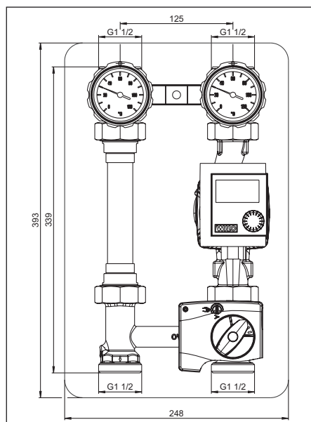
Fig. 6 Système de raccordement pour chaudières avec vanne mélangeuse à trois voies 180 mm DN25 avec robinet d'isolement à tournant sphérique (forme courte)
