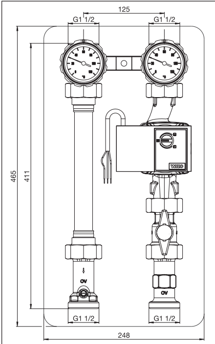
Fig.3 Sistema di collegamento caldaia 180 mm DN25 con valvola a sfera prima del circolatore (versione lunga)
