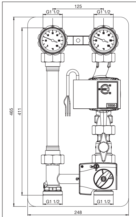
Abb. 4 Pumpengruppe mit 3-Wege-Mischhahn, 180 mm DN25 mit Pumpenkugelhahn (lange Bauform)
