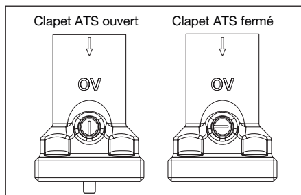
Fig. 7 Position clapet ATS
