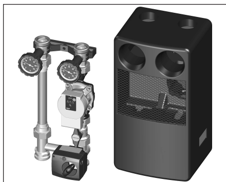
Fig. 1.1 Système de raccordement pour chaudières avec vanne mélangeuse à trois voies DN25 (En fonction du modèle, livré avec ou sans grille de ventilation).
