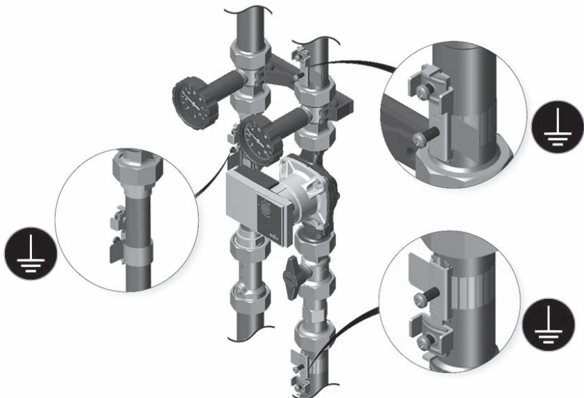
Abb. 26 Schutzpotentialausgleich/Erdung einer Installation mit Metall Verrohrung
