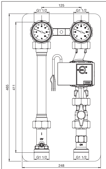
Abb. 3 Pumpengruppe 180 mm DN25 mit Pumpenkugelhahn (lange Bauform)
