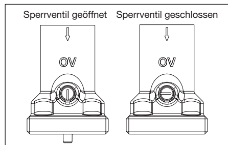
Abb. 7 Stellung Schwerkraftsperre
