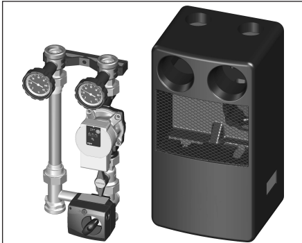
Fig. 1 Sistema di collegamento caldaia con valvola miscelatrice a tre vie DN25. (Fornitura possibile con o senza griglia di aerazione, a seconda della versione).
