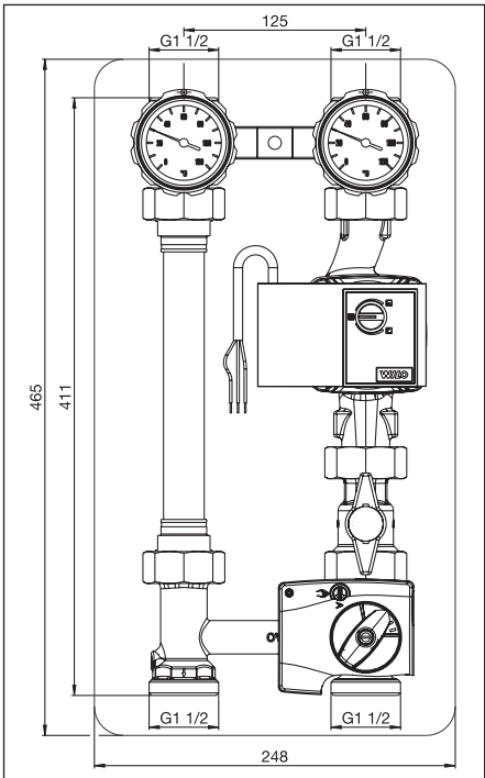
Fig.4 Sistema di collegamento caldaia con valvola miscelatore a tre vie 180 mm DN25 con valvola a sfera prima del circolatore (versione lunga)
