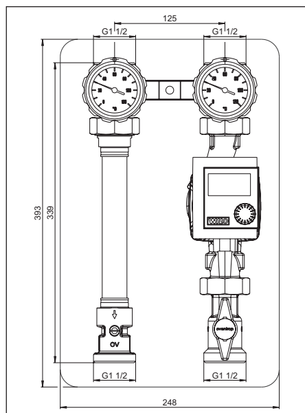
Fig.5 Sistema di collegamento caldaia 180 mm DN25 con valvola a sfera prima del circolatore (versione corta)
