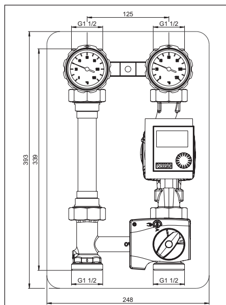
Fig.6 Sistema di collegamento caldaia con valvola miscelatore a tre vie 180 mm DN25 con valvola a sfera prima del circolatore (versione corta)
