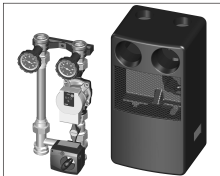
Abb. 1 Pumpengruppe mit 3-Wege-Mischhahn DN25 (Auslieferung je nach Ausführung mit oder ohne Lüftungsgitter möglich).
